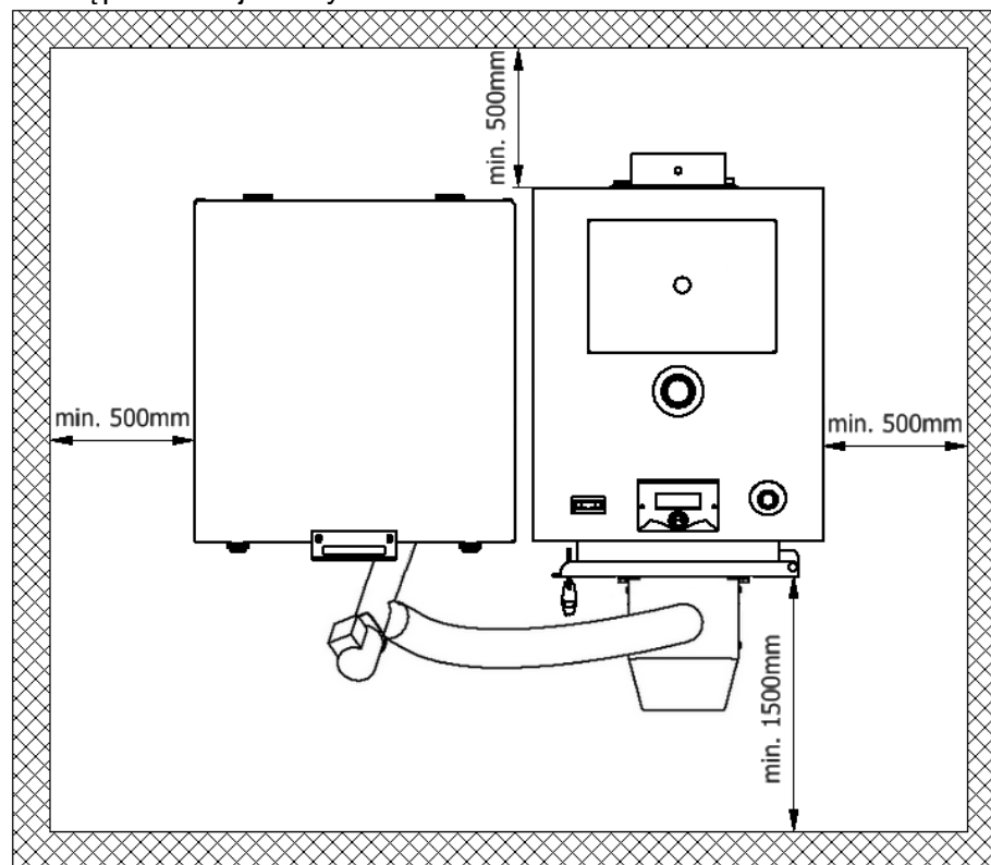
Rys 3. Ustawienie kotła KAMEN w pomieszczeniu kotłowni.
