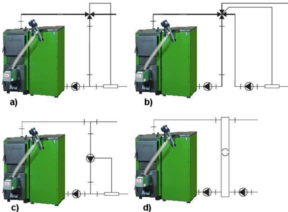
Rys. 4. Zalecane schematy połączenia kotła KAMEN z instalacją grzewczą: a) z zaworem trójdrożnym; b) z zaworem czterodrożnym; c) z pompą przewałową; d) ze sprzętem hydraulicznym
